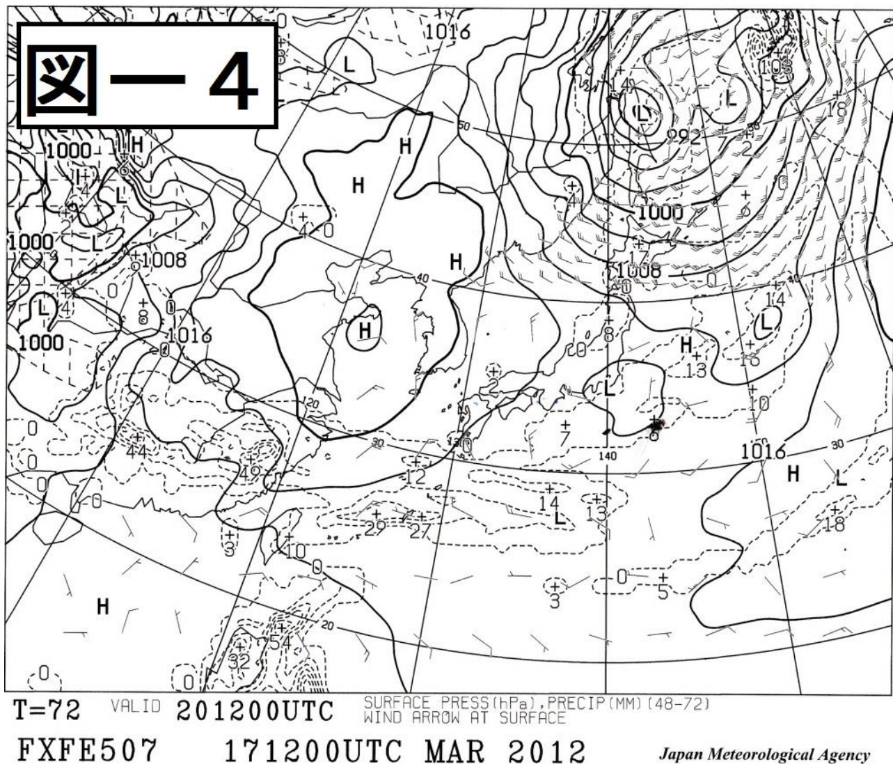
(図-4 極東地上気圧、風、降水量予想図 20日21時)
