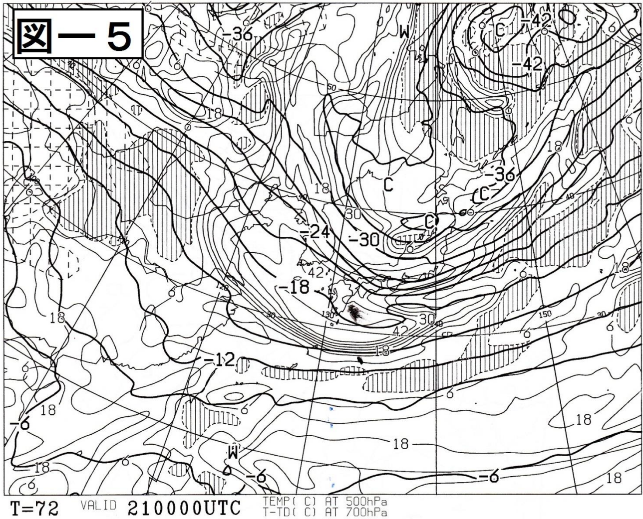
(図－5 500hPa 気温、 700hPa 湿数予想図 21 日 09 時)
