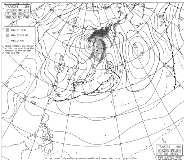
(地上予想天気図 18日21時)
