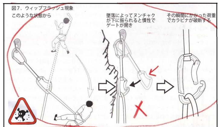
(本図引用＝菊池敏之著「最新アルパ インクライミング」、下図も同様)
